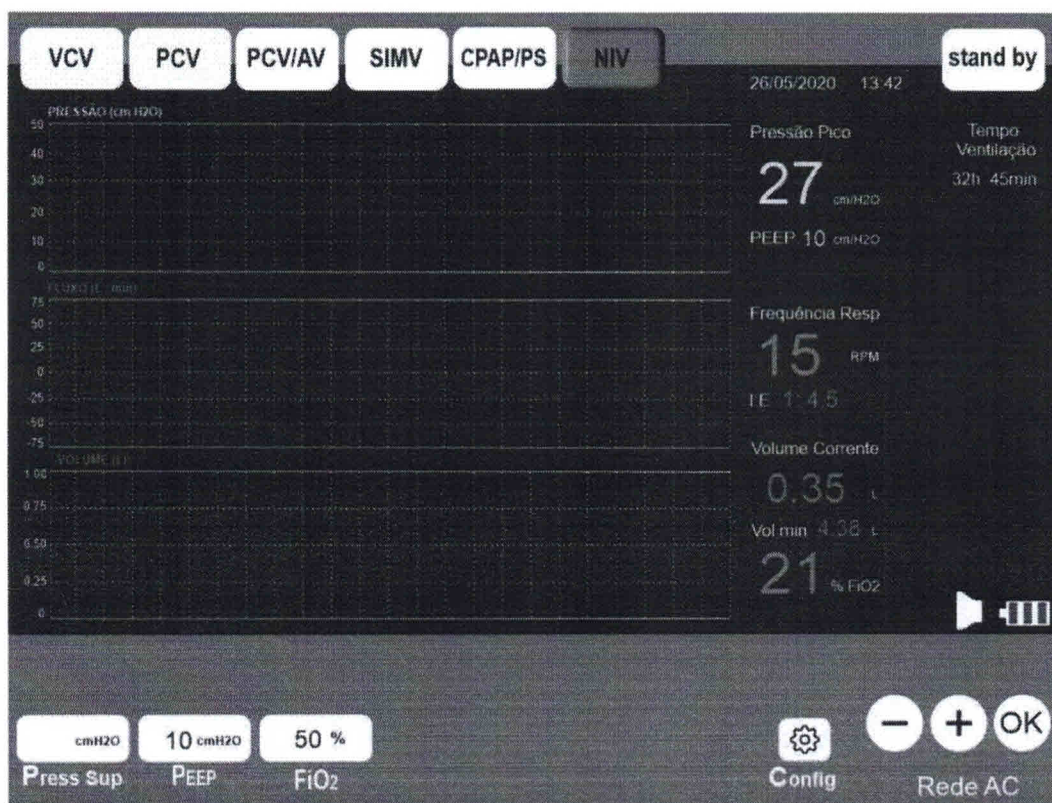
Figura 6: TELA NIV - VENTILAÇÃO NÃO INVASIVA
