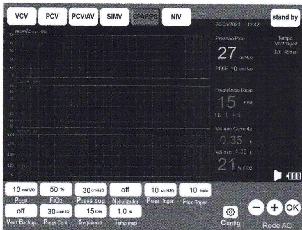
Figura 5: TELA CPAP/PS - VENTILAÇÃO COM PRESSÃO CONTÍNUA EM VIAS AÉREAS / VENTILAÇÃO COM PRESSÃO DE SUPORTE
