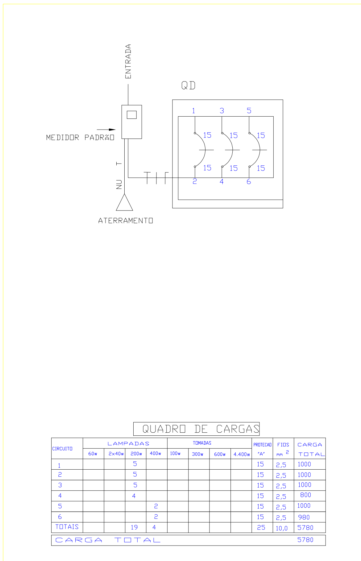
PLANTA LOCAÇÃO/ ELETRICO ESC.: 1/100
