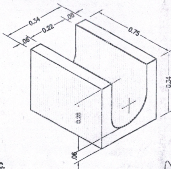
BLOCO DE ANCORAGEM PRÉ-MOLDADO PARA TIL DE PASSAGEM DN150 À DN200
