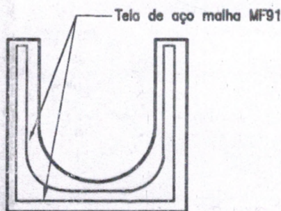
CORTE TRANSVERSAL DO BLOCO DE ANCORAGEM P/ TIL DE PASSAGEM - S/ESC.
