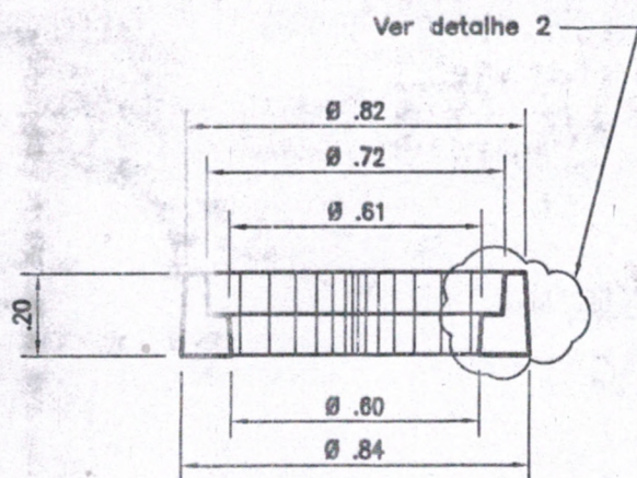
GUARNIÇÃO DO TAMPÃO EM CONCRETO ARMADO ESC. 1:10
