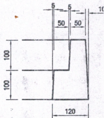
DETALHE 2 - SEM ESC. (Dimensões em milímetro)
