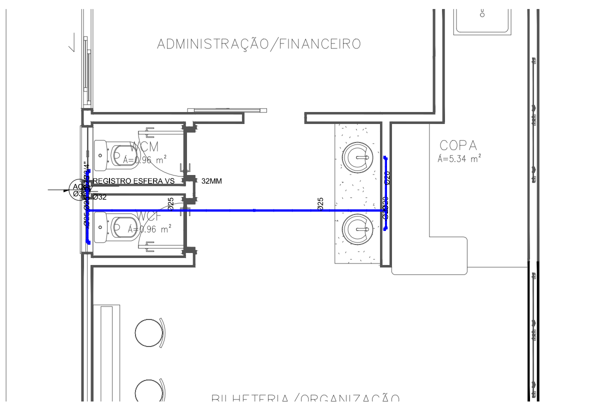
PLANTA INST. DETALHE 2 ESCALA 1/50
