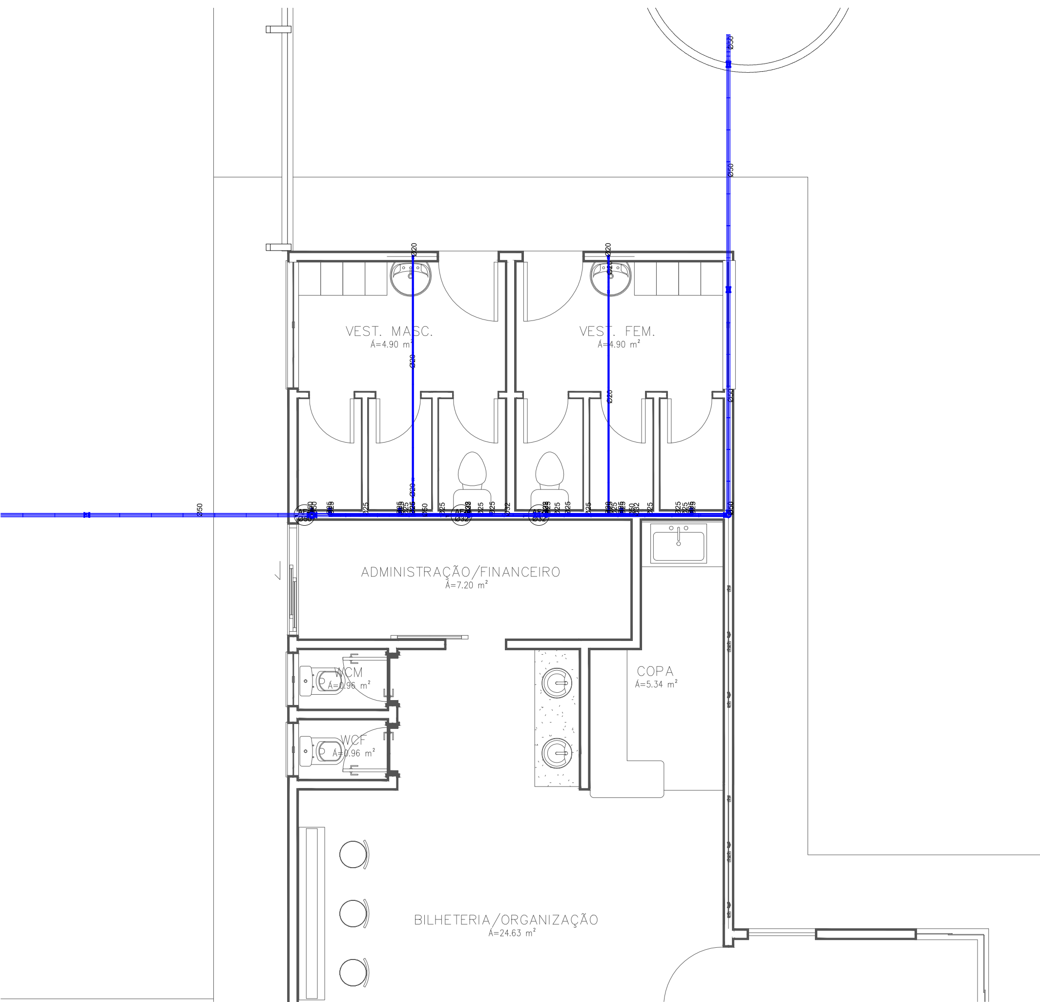
PLANTA INST. DETALHE 3 ESCALA 1/50
