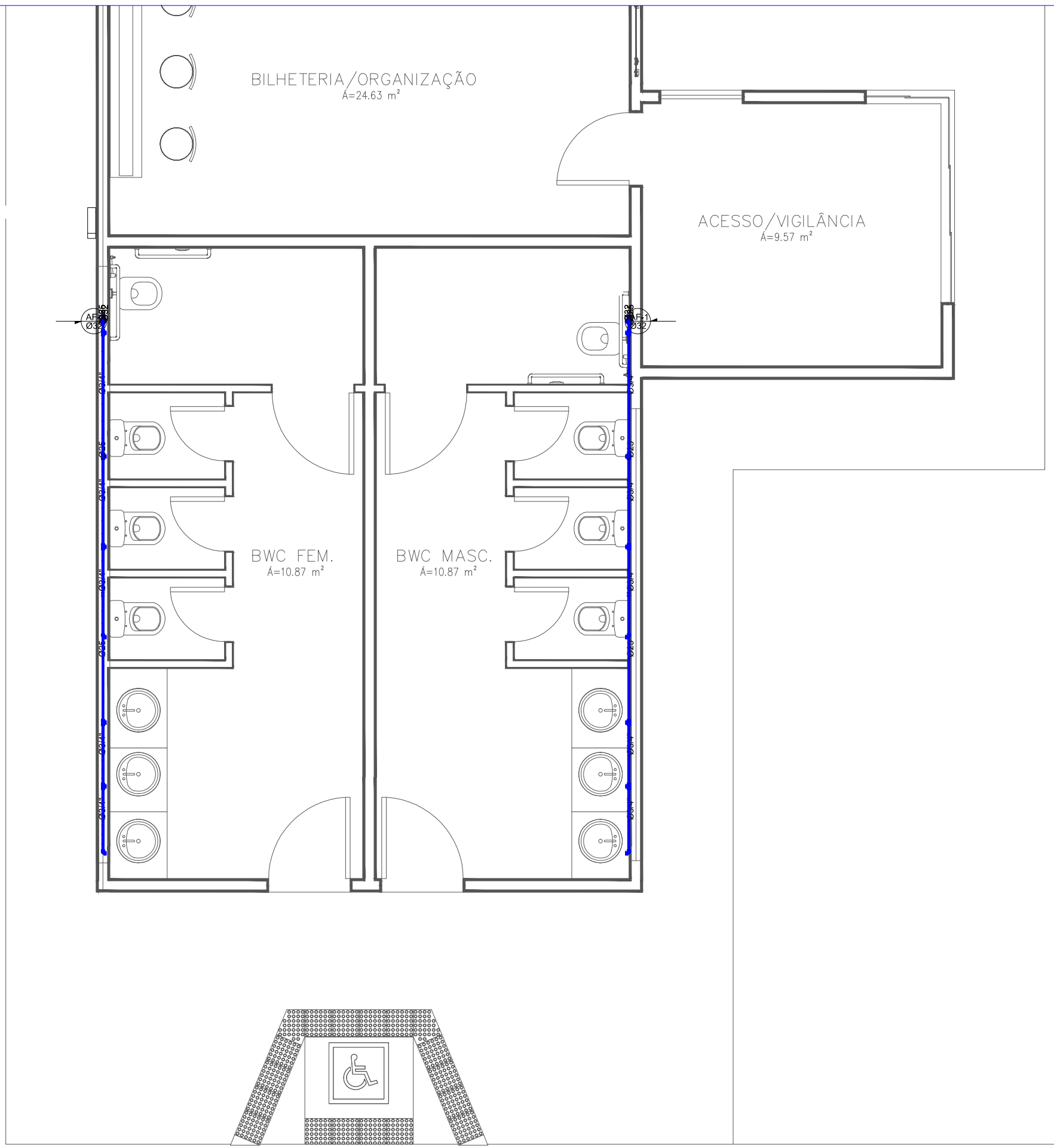
PLANTA INST. DETALHE 1 ESCALA 1/50
