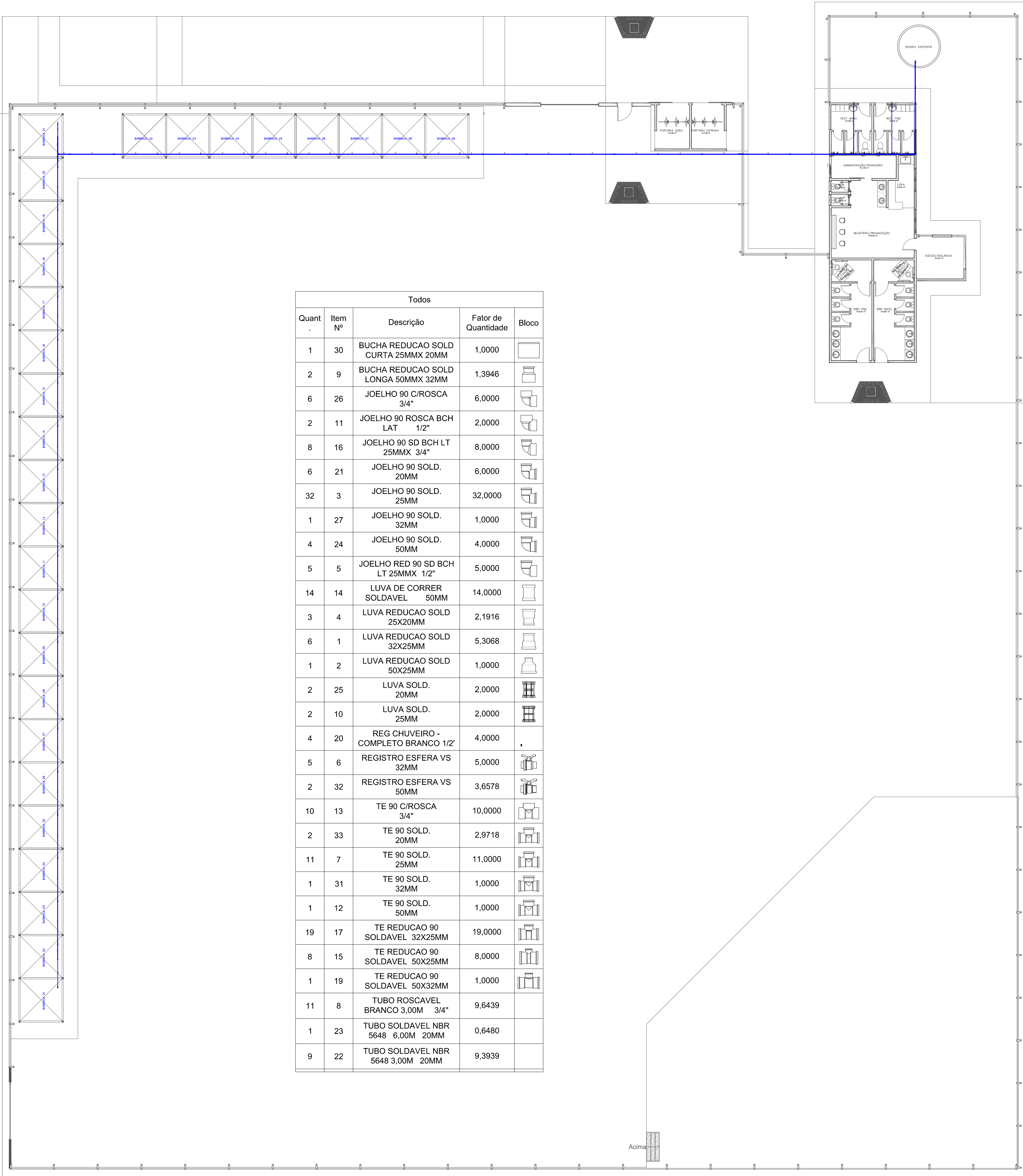
PLANTA DE INSTALAÇÃO GERAL ESCALA 1/150
